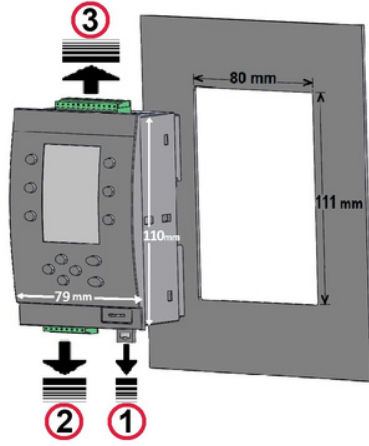
Şekil - 4 GSR-T panel montaj
