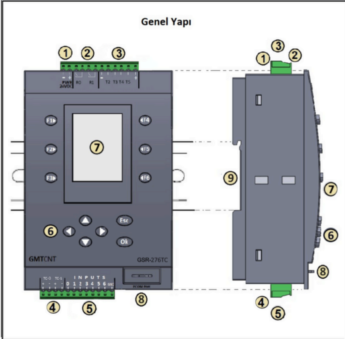
Şekil - 1 Cihazın yapısı
