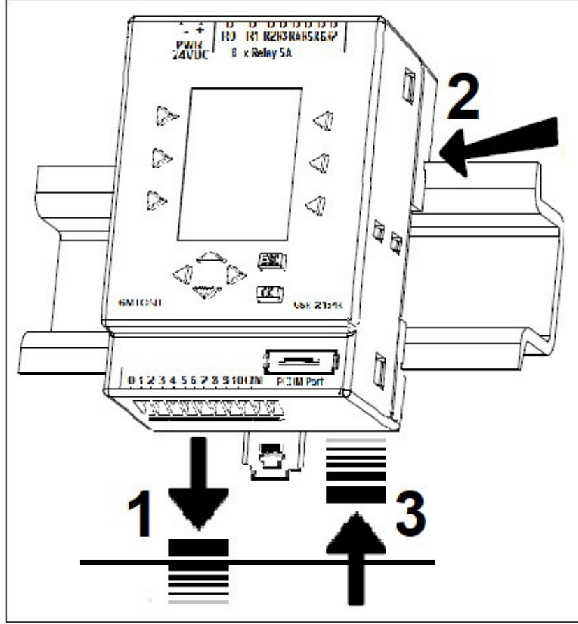
Şekil - 3 GSR-T DIN ray montaj
