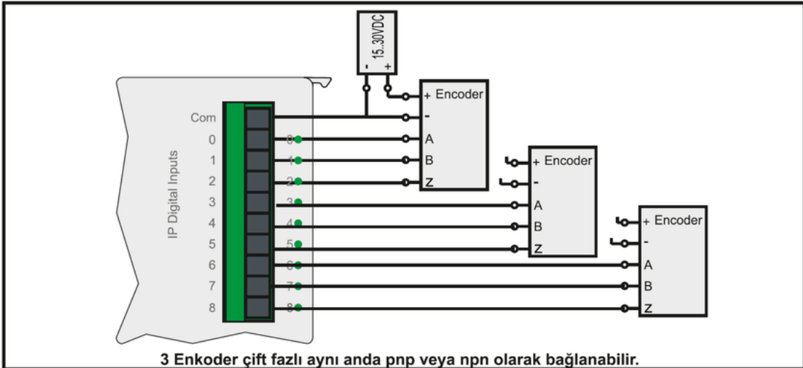
3 Encoder çift fazlı aynı anda npn veya pnp olarak bağlanabilir.
