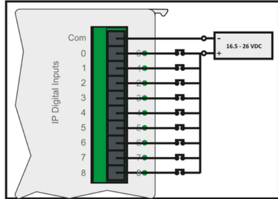
Girişlere kuru kontak bağlanması. pnp
